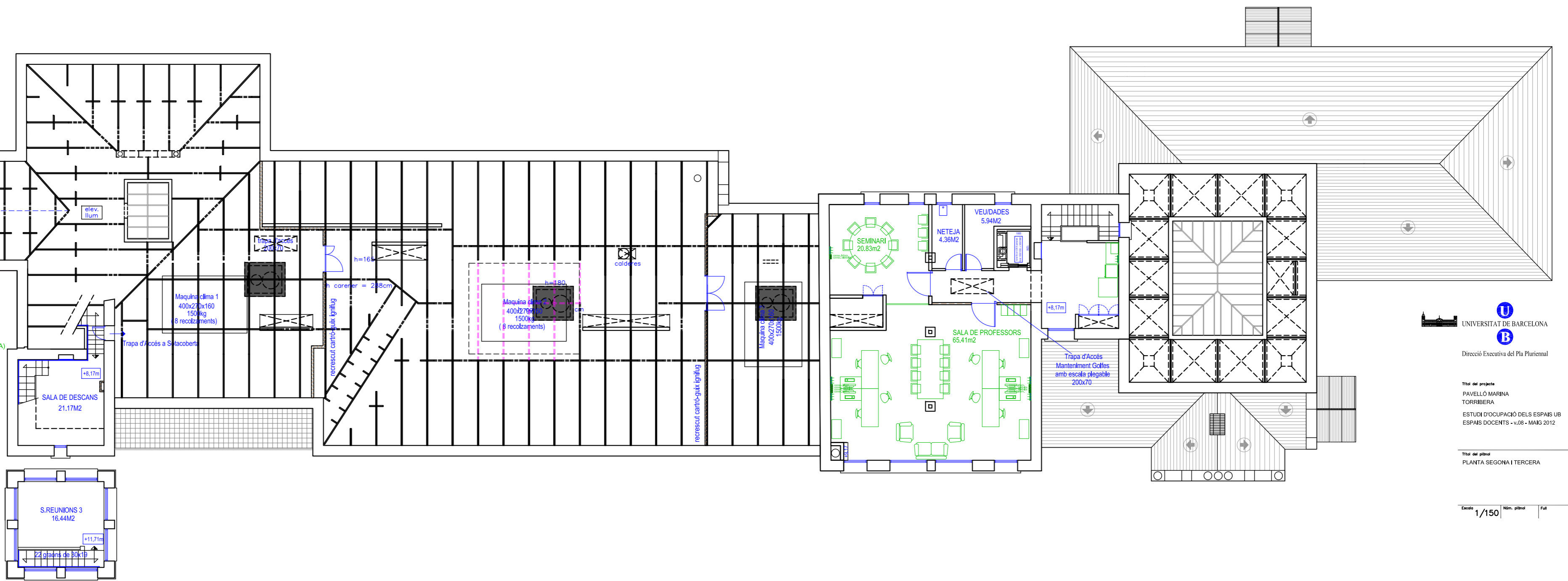
PLANTA SEGONA I TERCERA E:1/150
