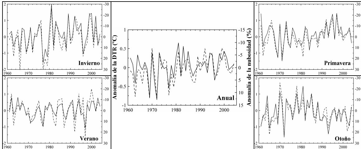
Fig. 1: Evolución anual y estacional de la DTR (línea continua) y la nubosidad total (discontinua) en España (1961-2004). La escala de la segunda aumenta hacia abajo.
