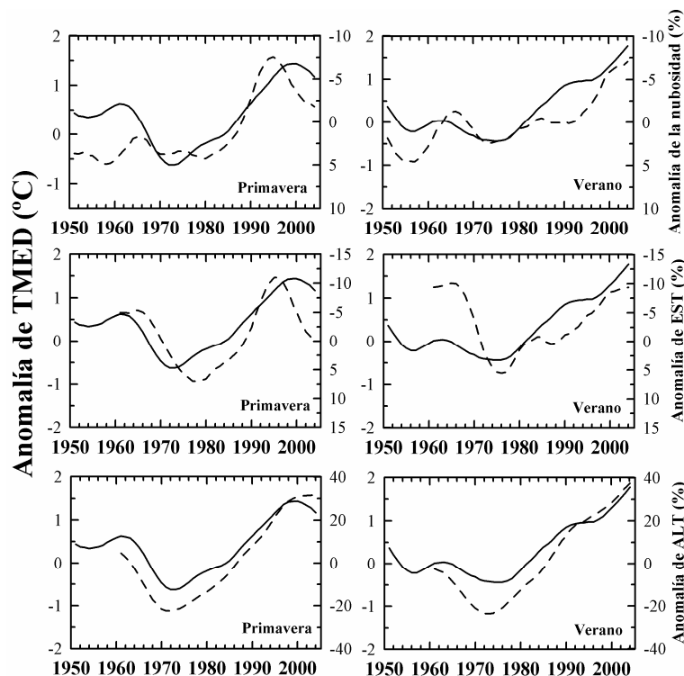
Fig. 3: Evolución primaveral (izquierda) y estival (derecha) de la TMED (línea continua) y la nubosidad total (fila superior), y familias de nubes EST (fila media) y ALT (fila inferior) en España (1951-2004). Nótese que sólo se muestran los valores ya suavizados por el filtro de paso bajo, que las series de EST y ALT están limitadas al período 1961-2004, y que las escalas de la nubosidad total y EST aumentan hacia abajo.
