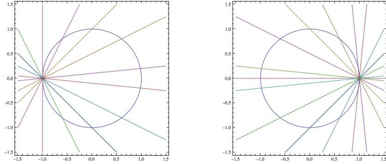
FIGURA 3: Rectes mòbils \mathcal{L}_1 (a esquerra) i \mathcal{L}_1^* (a dreta).
