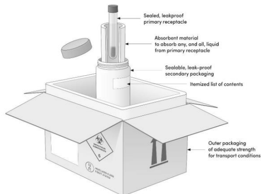
Figura 1: Exemple de triple envàs per una substància de Categoria A, seguint les instruccions d'embalatge P620.
