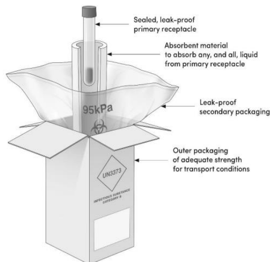
Figura 2: Exemple de triple envàs per una substància de Categoria B, seguint les instruccions d'embalatge P650.
