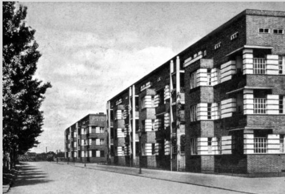
Berlin. Siedlung Schillerpark, 1924- 1930. Bruno Taut
