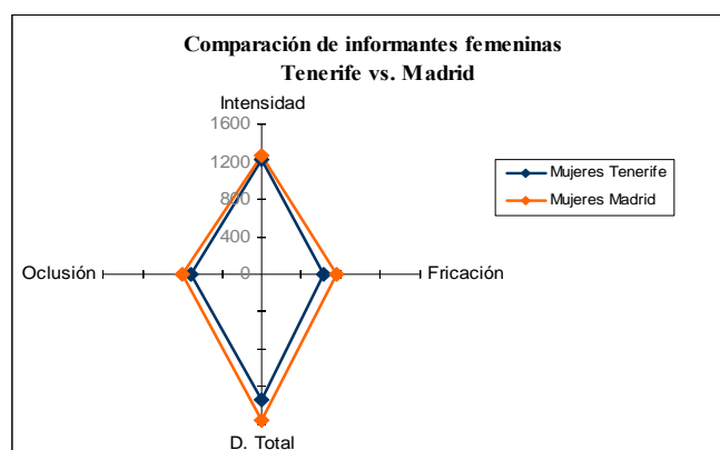
Figura 4. Comparación de duraciones e intensidad de [\hat{t}] entre mujeres de Tenerife y de Madrid.
