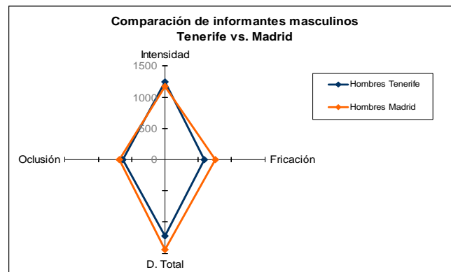
Figura 3. Comparación de duraciones e intensidad de [tʃ] entre hombres de Tenerife y de Madrid.
