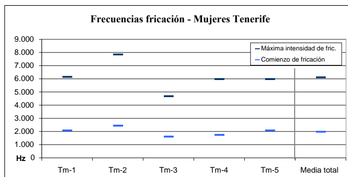
Figura 7. Frecuencias en Hz de comienzo y de máxima intensidad de fricación de [\hat{t}] de mujeres de Tenerife.
