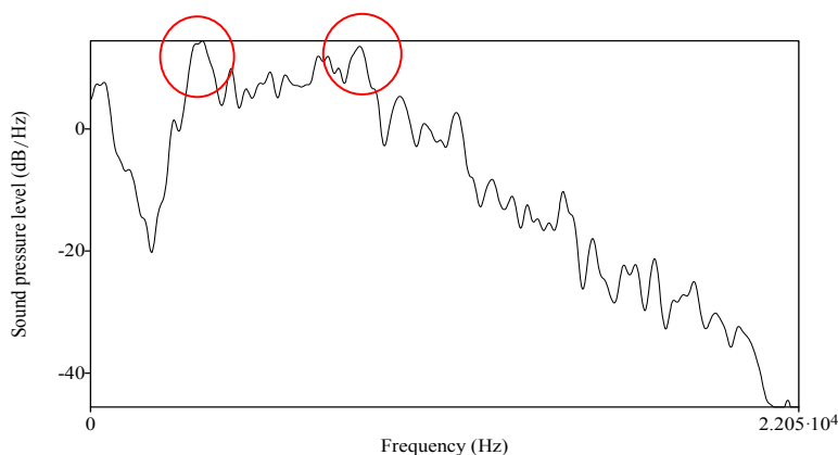
Figura 1. Suavizado de corte espectral de [o't̪o] en Th-3 Rep. 3.
