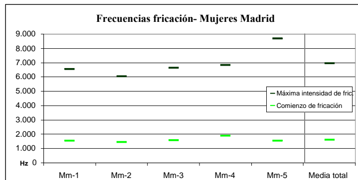
Figura 8. Frecuencias en Hz de comienzo y de máxima intensidad de fricación de [tʃ] de mujeres de Madrid.
