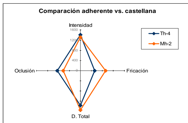
Figura 2. Comparación entre resultados de [t̪] de los informantes Th-4 y Mh-2.
