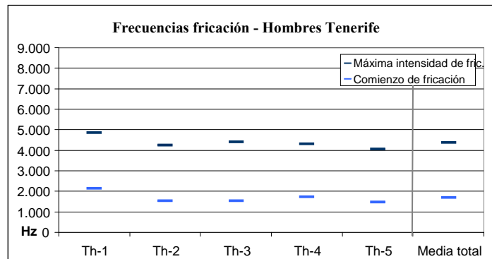
Figuras 5. Frecuencias en Hz de comienzo y de máxima intensidad de fricación de [tʃ] de hombres de Tenerife.
