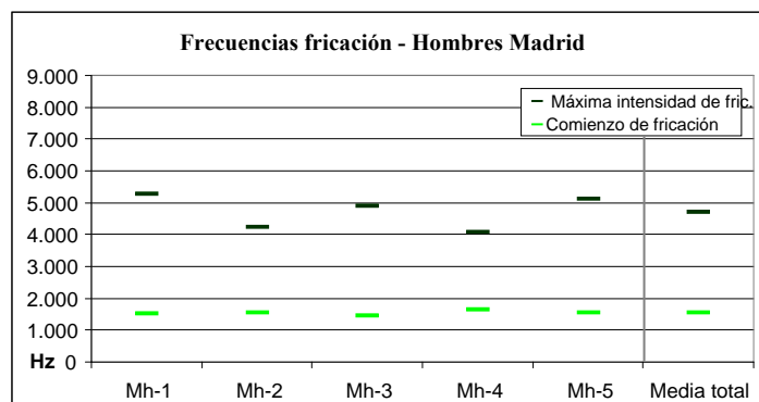
Figuras 6. Frecuencias en Hz de comienzo y de máxima intensidad de fricación de [tʃ] de hombres de Madrid.
